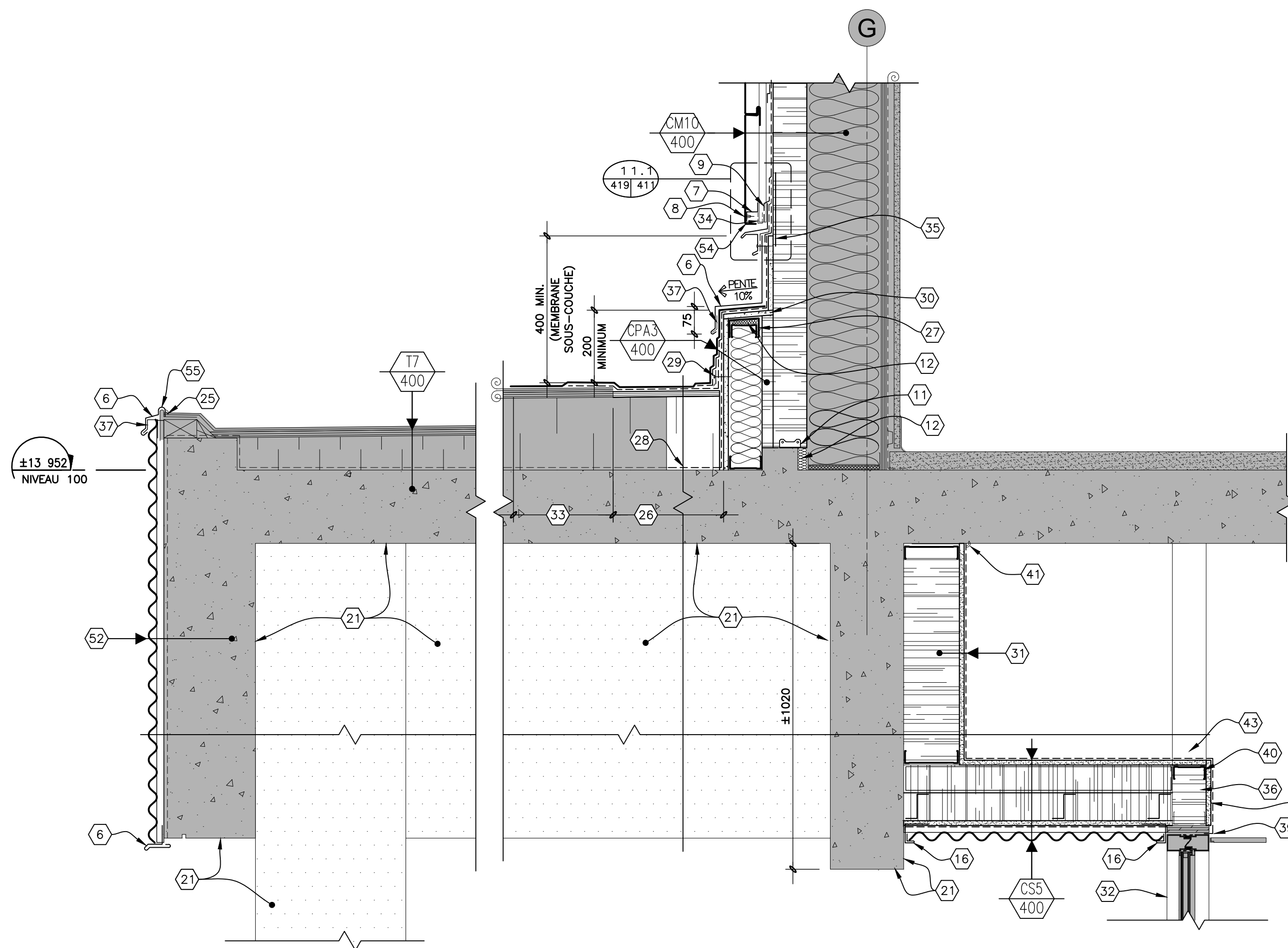
DÉTAIL TYPE MARQUISE 1:10mm (ENTRÉE PRINCIPALE)
